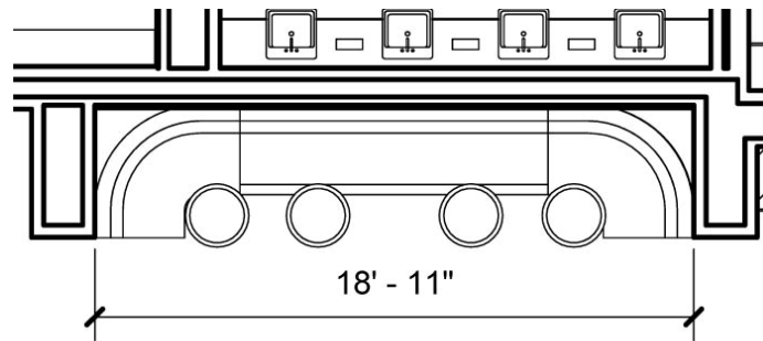
Plan (NTS)
